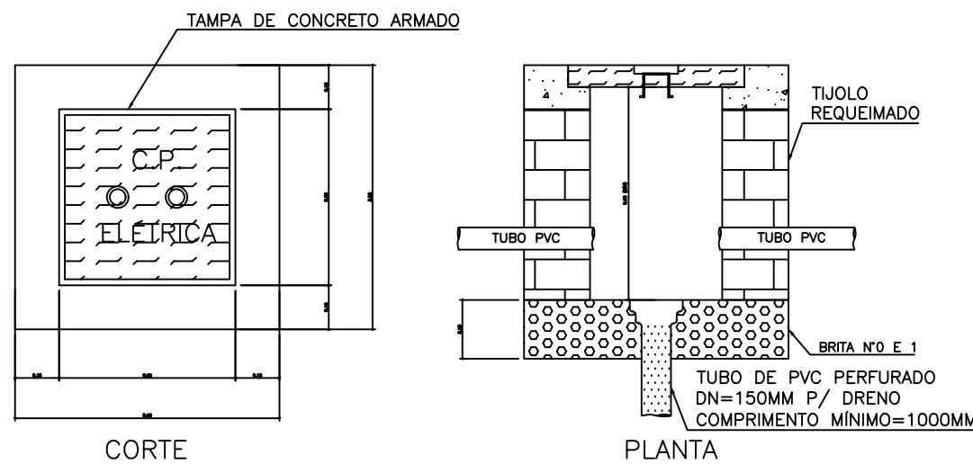
DETALHE DA CAIXA DE PASSAGEM SUBTERRÂNEA
